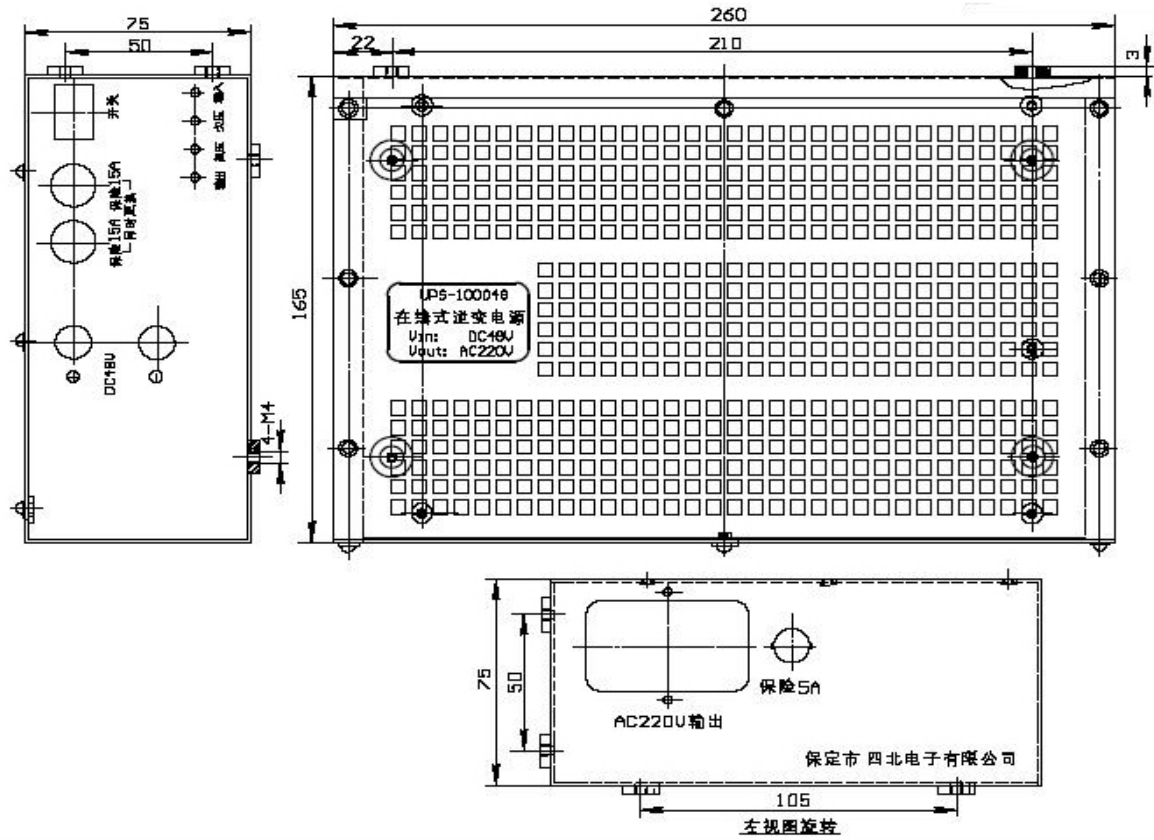
安装尺寸及输出输入示意图
